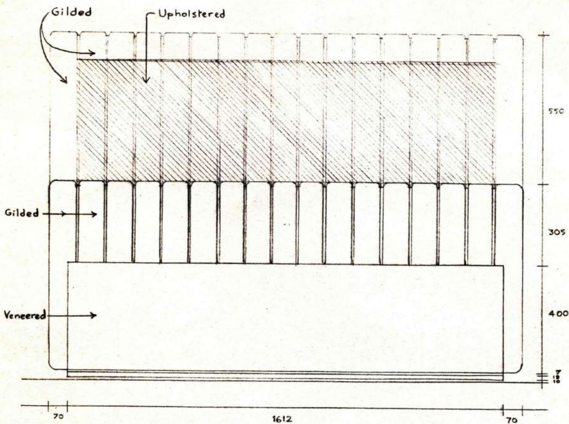
ELEVATION B
